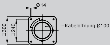
Bodenbefestigung
