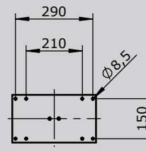
Bodenbefestigung
