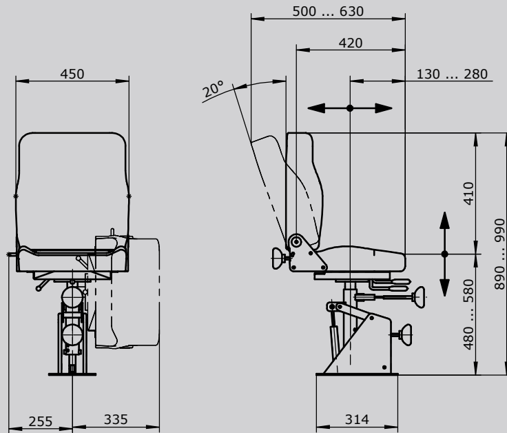
Bodenbefestigung
