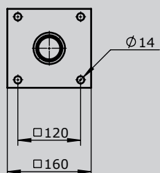
Bodenbefestigung
