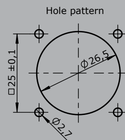
Actuator KBAD 1690
