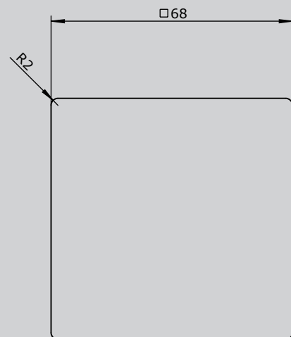
Einbauöffnung
